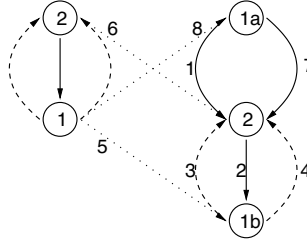
Fig. 3. Memoized Corecursion
